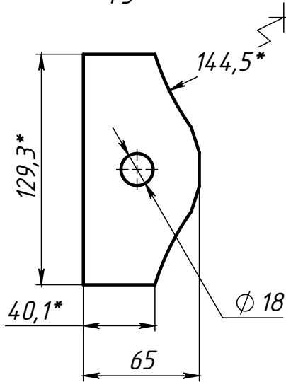
Поз.6 (Ушко) развертка 1:3
