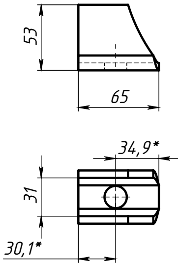
Поз.6 (Ушко) 1:3
