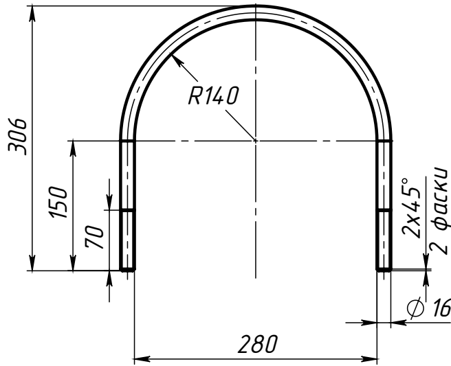
Поз.5 (Хомут)
