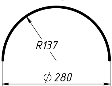
Поз.4 (Прокладка)
