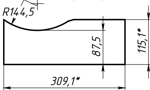
Поз.2 (Угольник) развертка
