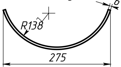
Поз.3 (Подушка)
